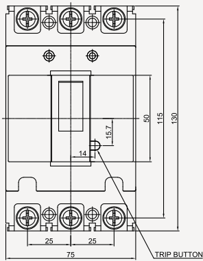
◆ 3 POLE
