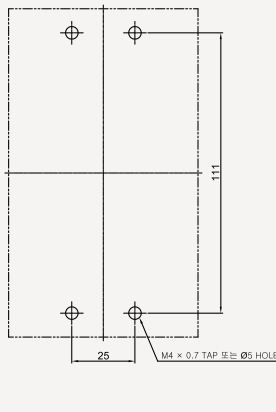
◆ 부착 HOLE
