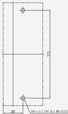
◆ 부착 HOLE
