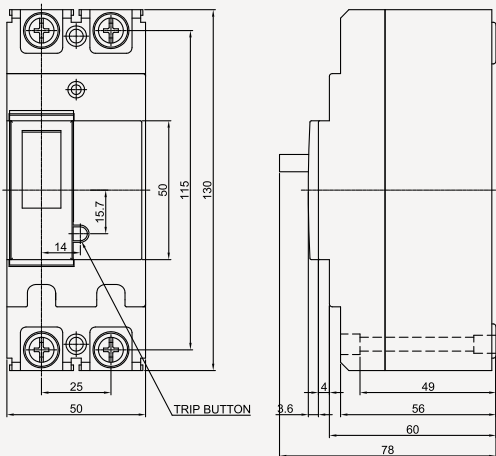
◆ 2 POLE
