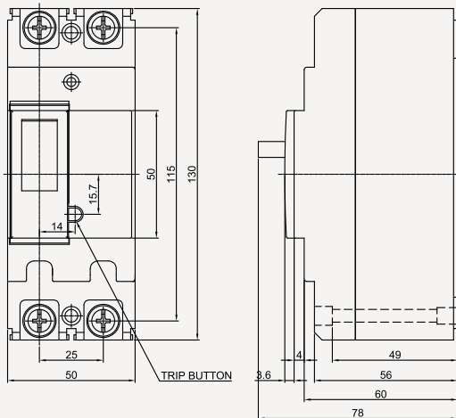
◆ 2 POLE
