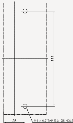
◆ 부착 HOLE
