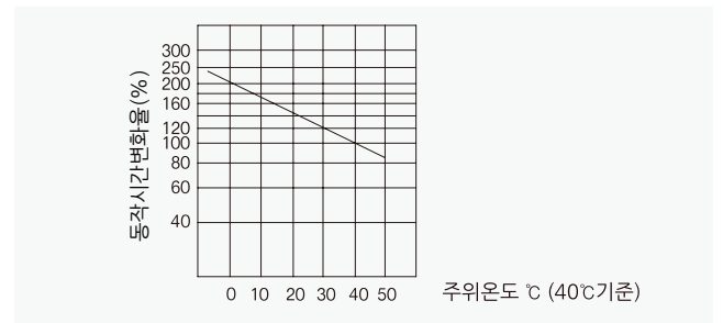
온도보정곡선
