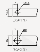
◆ 접속 도체 가공도
