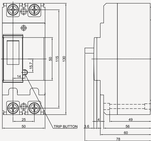
◆ 2 POLE
