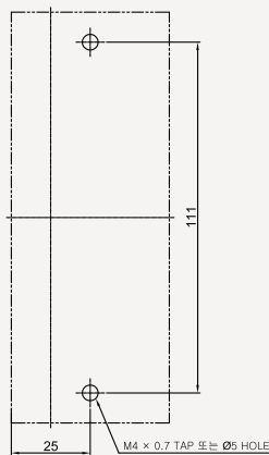
◆ 부착 HOLE
