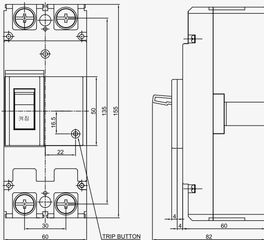
◆ 2 POLE
