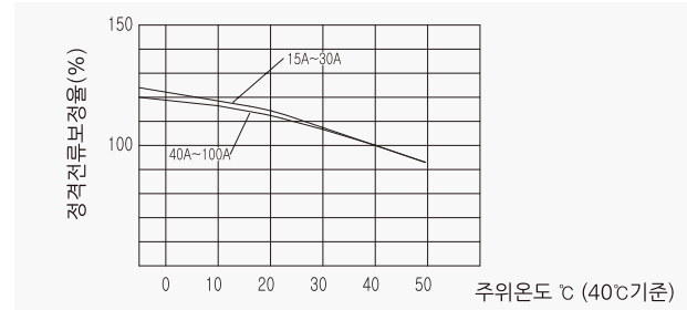
온도보정곡선
