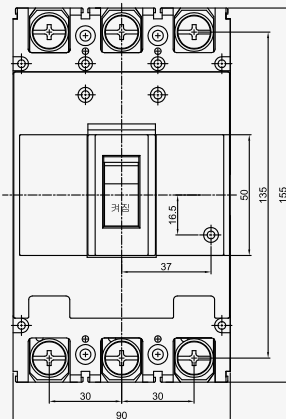
◆ 3 POLE
