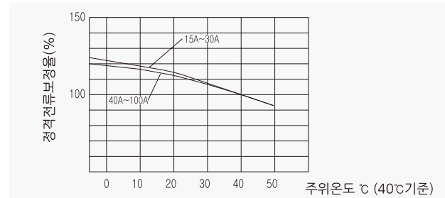
온도보정곡선
