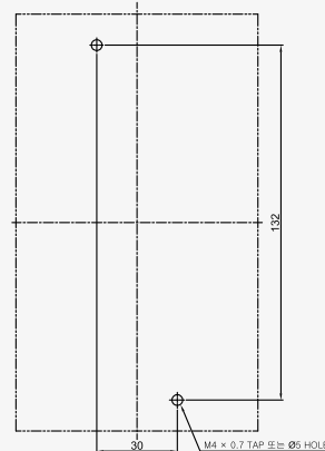
◆ 부착 HOLE
