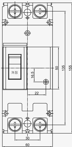
◆ 2 POLE
