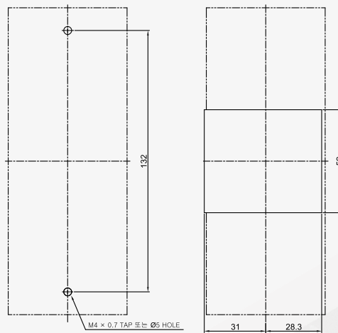
◆ 부착 HOLE
