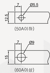
◆ 접속 도체 가공도
