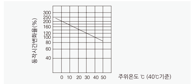
온도보정곡선
