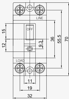
◆ 2 POLE
