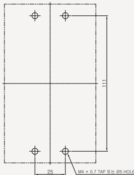
◆ 부착 HOLE
