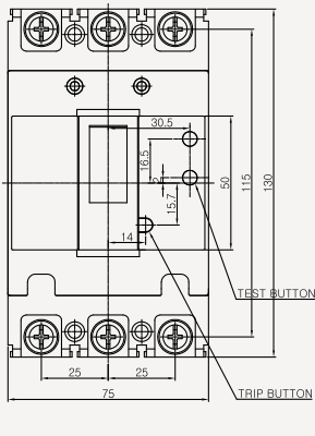
◆ 3 POLE
