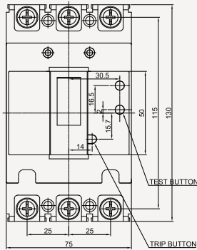
◆ 3 POLE
