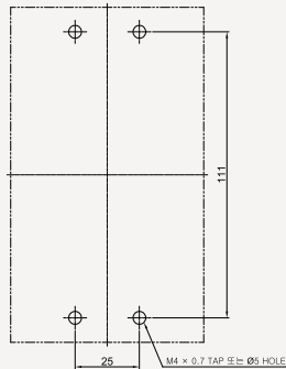
◆ 부착 HOLE
