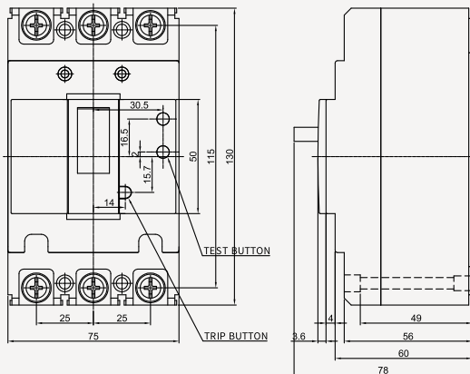
◆ 3 POLE
