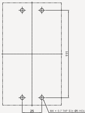
◆ 부착 HOLE
