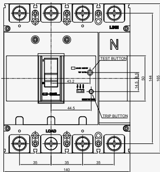
◆ 4 POLE
