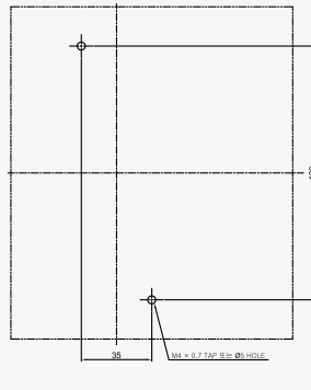
◆ 부착 HOLE
