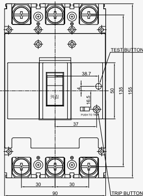
◆ 3 POLE
