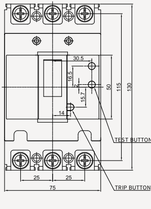
◆ 3 POLE
