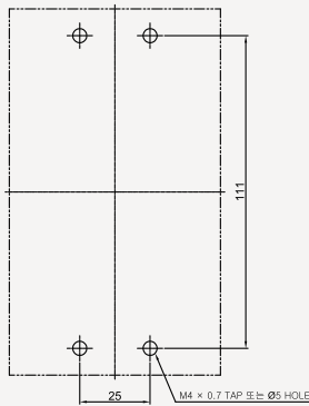
◆ 부착 HOLE
