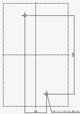
◆ 부착 HOLE
