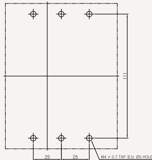
◆ 부착 HOLE
