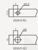
◆ 접속 도체 가공도
