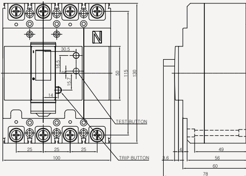
◆ 4 POLE
